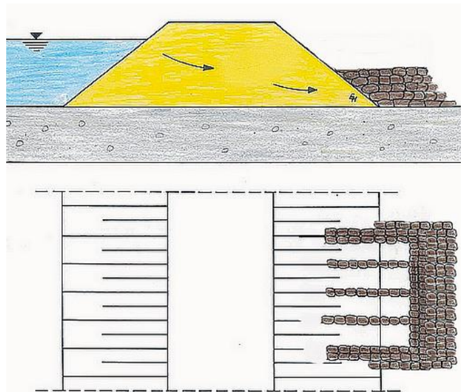
Bild 20: Prinzipskizze Kammkade
