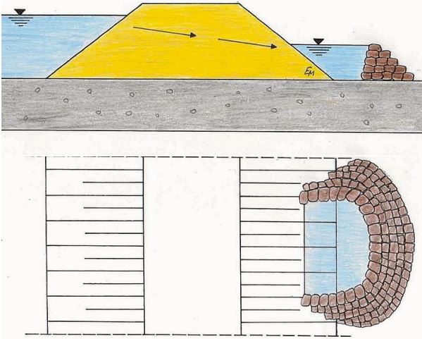
Bild 19: Prinzipskizze Quellkade
